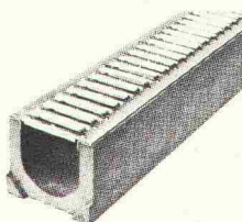
FASERFIX-Rinne mit Klemmrost (6 t RD)
