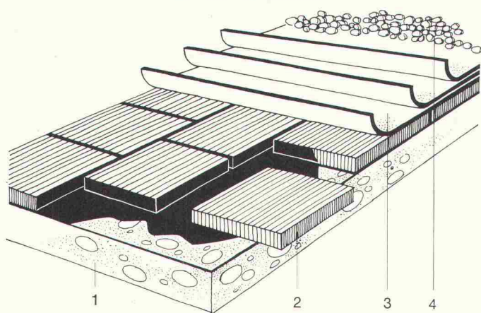
1. Tragende Konstruktion 2. FOAMGLAS® 3. Dachhaut 4. Kiesschüttung
