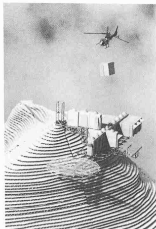
Unten links: Montage der Tragkonstruktion mit Helikopter Unten rechts: Montage der Raumzellen mit Helikopter
