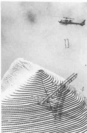
Unten links: Montage der Tragkonstruktion mit Helikopter Unten rechts: Montage der Raumzellen mit Helikopter
