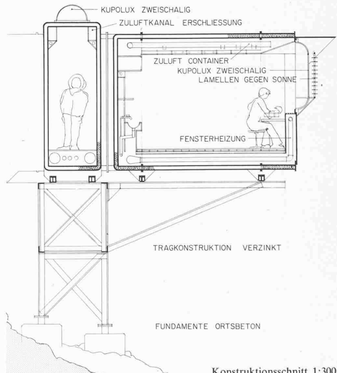
Konstruktionsschnitt 1:300
