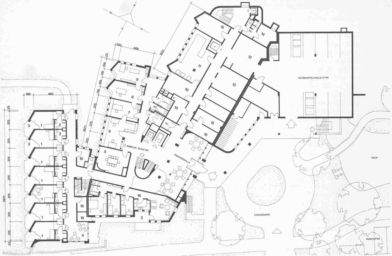
Grundriss Erdgeschoss 1:450. 1 Zimmer, 2 Dusche/WC, 3 Balkon, 4 Aufenthalt, 5 Sitzungsraum/Bibliothek, 6 Sekretariat, 7 Heimleitung, 8 Hausbeamtin, 9 Arzt/Krankenschwester, 10 Container, 11 Wäscherei, 12 Leergut, 13 Kühlraum, 14 Ruheraum, 15 Geräte/Putzraum, 16 Wohnung Hauswart
