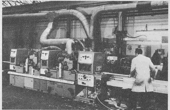
Die neue Holzbearbeitungsmaschine FBN 230 der Firma Wadkin bearbeitet dünnes Holz mit Geschwindigkeiten bis zu 100 m/Min.
