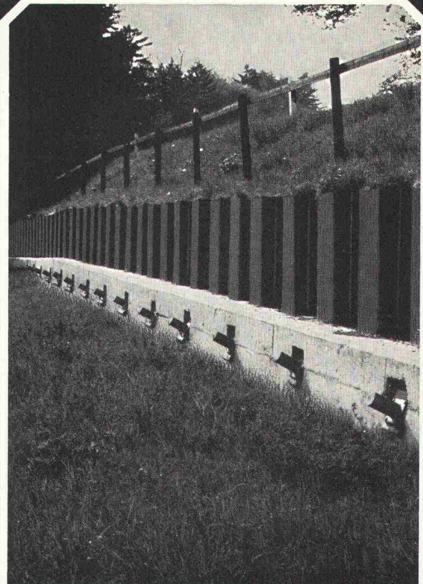
Rutschsanierung Hüntwangen
