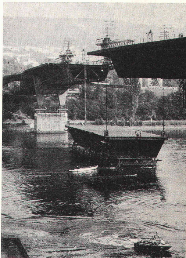
Hochheben des 650 Mp schweren Mittelteils der Horschheimer Rheinbrücke bei Koblenz.
