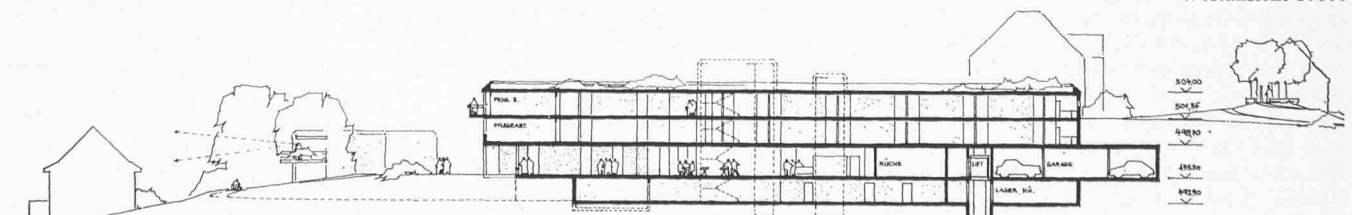
Schnitt 1:800
