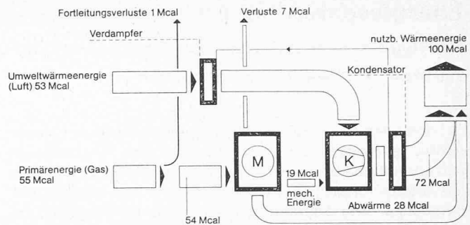
Energieflussbild der Gas-Wärmepumpe
