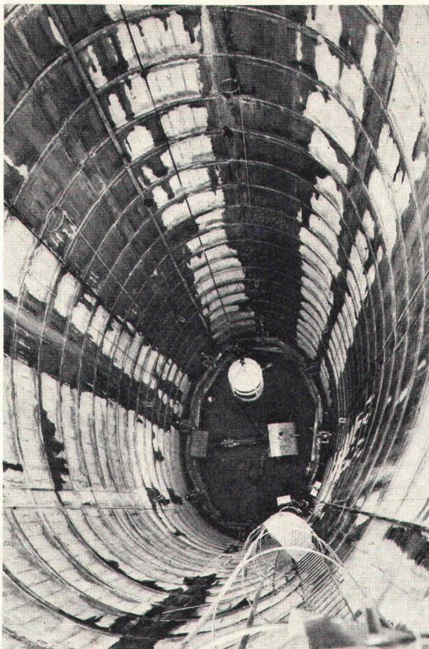
Blick in einen der ellipsenförmigen Gelenk- schächte (9.60 m/7.00 m).
