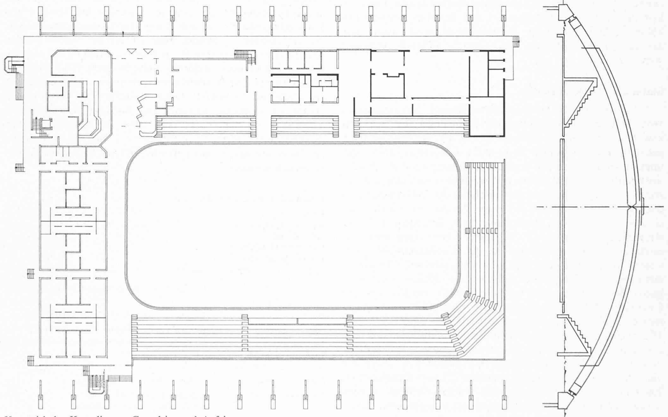
Kunsteisbahn Kreuzlingen. Grundriss und Aufriss
