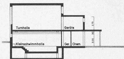
Schnitt durch Turnhalle und Schwimmhalle 1:450
