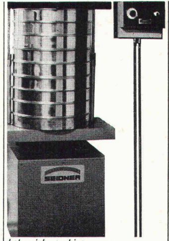
Laborsiebmaschine
