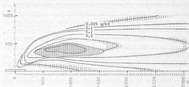
Rechnerische Darstellung der Orte gleicher Erhöhung der absoluten Feuchte durch den Betrieb eines Kühlsystems
