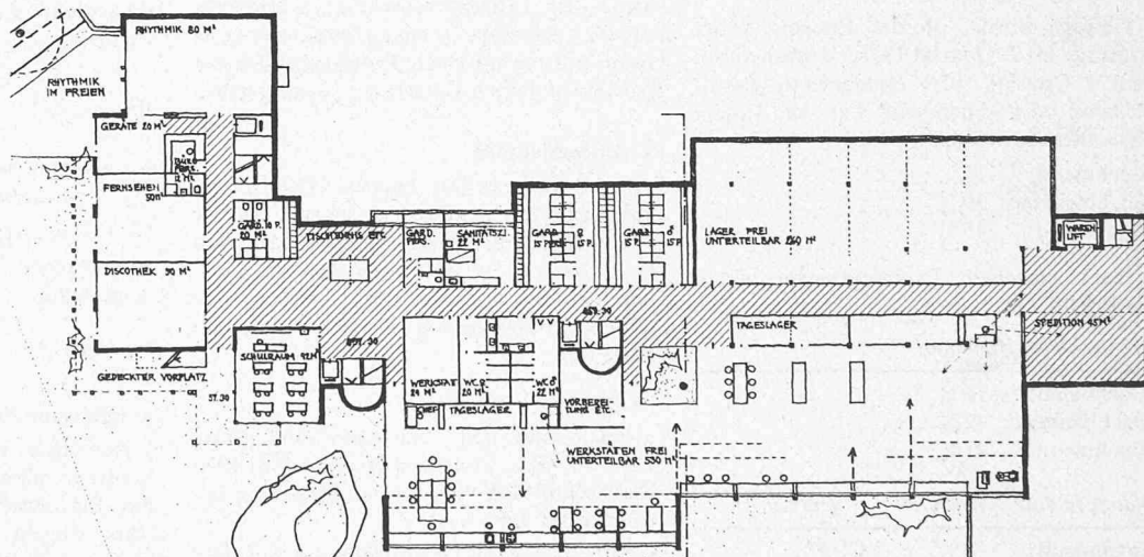
Grundriss Edgeschoss 1:600
