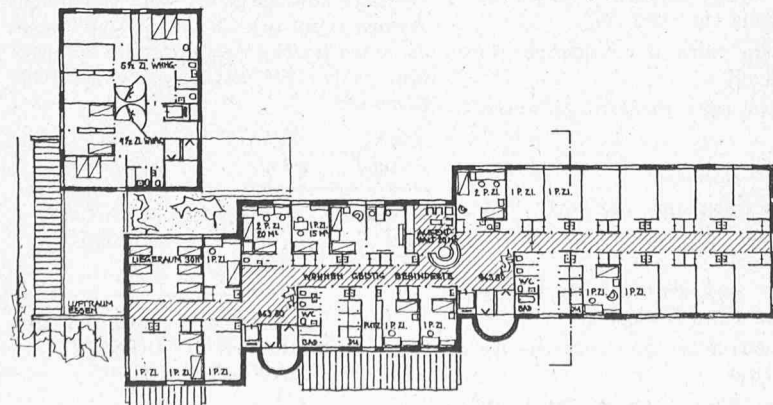
Grundriss 1. Obergeschoss 1:600
