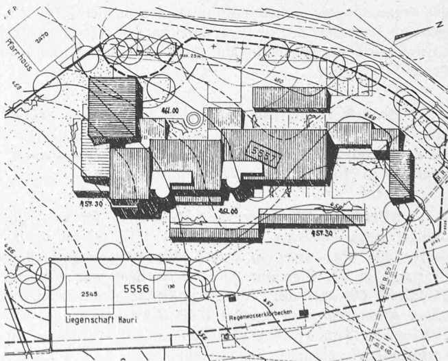
Lageplan 1:1200
