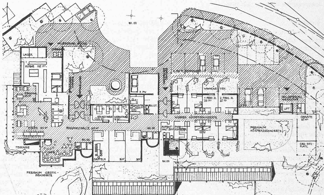
Grundriss Eingangsgeschoss 1:600
