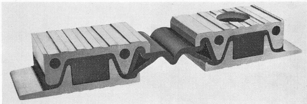
ELASTFUGE — eine vorgespannt verankerte, hochelastische Fahrwege aus Aluminium-Neopren Verbundelementen.
