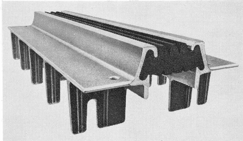
RIPPENFUGE — eine starr einbetonierte robuste Fahrwege aus feuerverzinktem Kugelgraphitguss.
