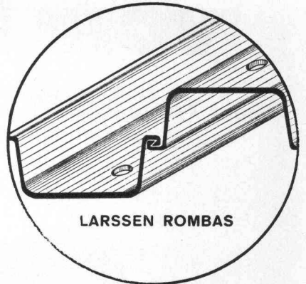
LARSEN ROMBAS Rampfpfähle LARSEN ROMBAS und unser Zubehör – Rammhauben, Eckprofile Omega und Delta, Ankermaterial und Dichtungsbänder – sind wertvolle Ergänzungen für das sichere und wirtschaftliche Gründungsverfahren LARSEN ROMBAS.
