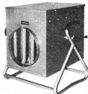
HATRA-Elektro-Heissluft-Gebläse für Raumheizung
