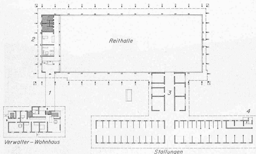
Grundriss Erdgeschoss 1:900. 1 Haupt- eingang, 2 Besucher- und Verwaltungs- räume (darüber Tribüne), 3 im Verbin- dungstrakt zwischen Stallgebäude und Reithalle die Betriebsräume (Sattelkam- mer, Schmiede, Werkstatt, Vorräte usw.), 4 Eingang zur Personalunterkunft im Dachgeschoss
