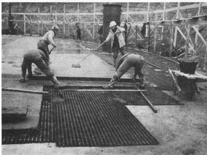
Bodendrainage Reaktorgebäude KKW Gösgen/Schweiz
