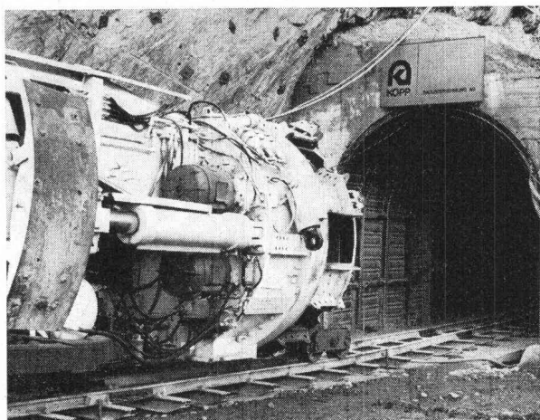
Einsatz einer Robbins-Streckenvortriebsmaschine für einen Kraftwerkstollen
