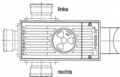
Primus 70 3fach gesicherter Kellerablauf gegen Rückstau
