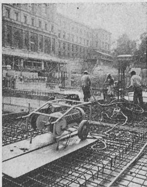
Einsatz von Laier Beton-Hochfrequenz-Vibratoren auf der Polytterasse
