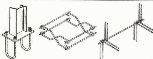
Befestigung von Leitholmen Felsenau-Wankdorfbrücken
