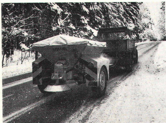
Salz- und Splittstreuer-Anhänger AMA-6H, Inhalt 750 l
