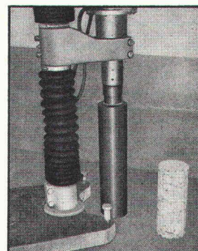
Leistungsfähige Bohrmaschine: Bohrleistung bis 250 mm Ø. (Neukonstruktionen für grössere Durchmesser in Bearbeitung.)
