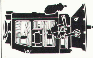
Getriebe SR 61
