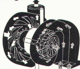
Abgasturbolader
