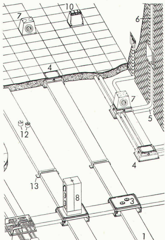
«teli-Flur» Installationssysteme
