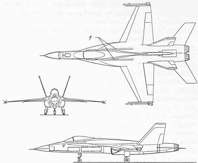
Dreiseitenansicht des Jagdflugzeuges Northrop YF-17. 1 Überströmschlitz.
