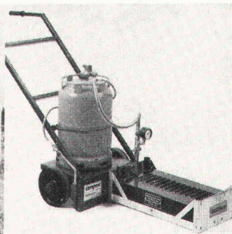
MILLARS Infrarot-Fugen- und Flächenheiz- geräte für Asphaltbeläge, fahr- bar und anbaubar an Fertiger
