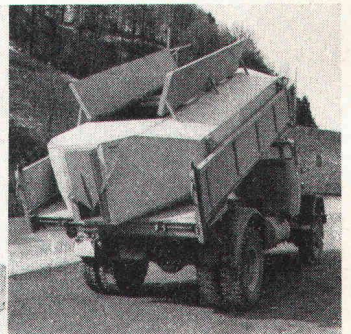
TIMPEX Warmhaltesilo für Belagsmisch- gut bei Handeinbau, Fassungs- vermögen ca 7 t
