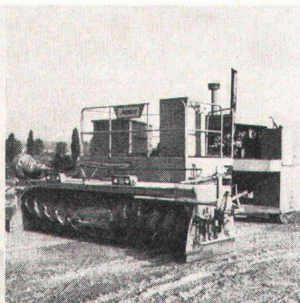
RAHCO Maschine zum Präzisionspla- nieren und zum Stabilisieren
