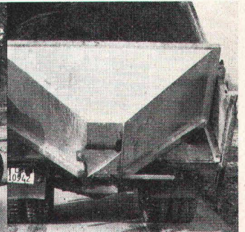
TIMPEX Auslauftrichter zum dosierten Abkippen von Belagsmischgut und Beton etc
