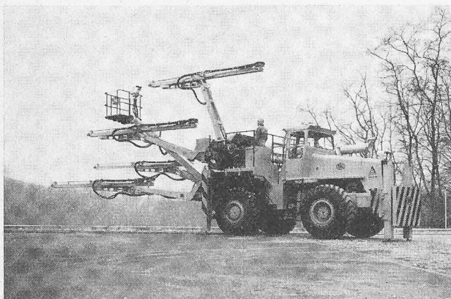
Vierarmiger SIG-Bohrwagen mit Ladkorb auf Knickgelenkfahrzeug, Type BAP 4-380 + L, mit Wirkungsfläche bis 47 m 2 Profilquerschnitt
