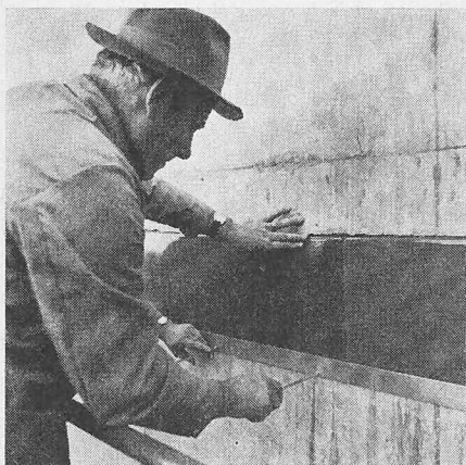
Die in Serie gefertigten Emailplatten werden auf der Baustelle in eine Beckenwandnische eingelegt und mit einem rostfreien Stahlprofil unten und oben fixiert
