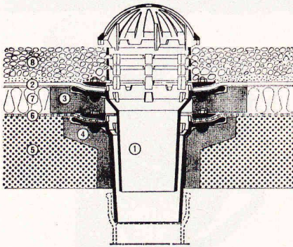
Kiesschüttdach, 2teilig
