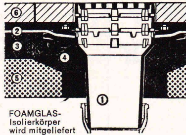
Dachterrasse, einteilig
