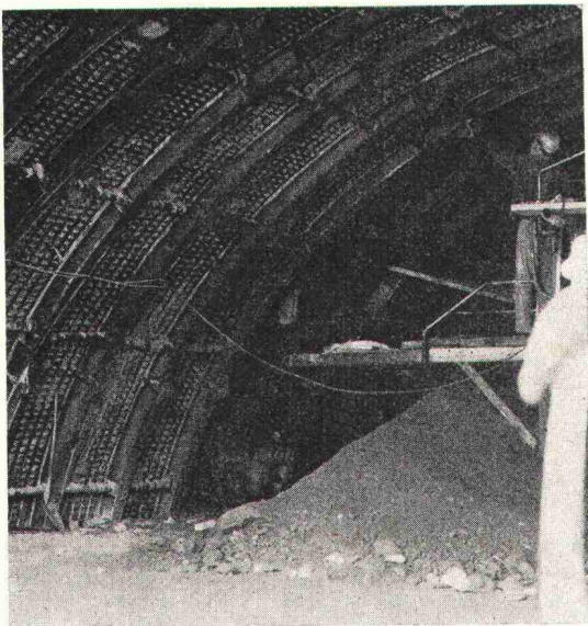
Tunnelauskleidung mit Schalungs- und Armierungsblechen Bernold®
