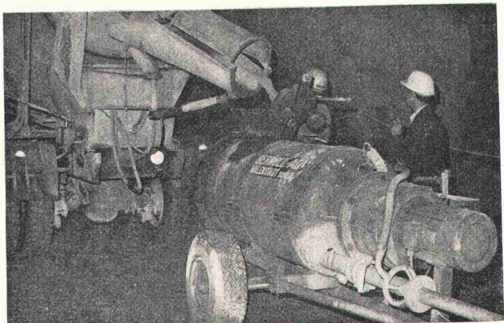
Betonpumpe Spiroret zum Fördern und Nassspritzen - die Pumpe mit der grossen Leistung
