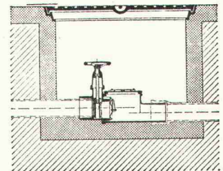
Rückstaudoppelpverschluss TRIPLEX für durchgehende Leitungen
