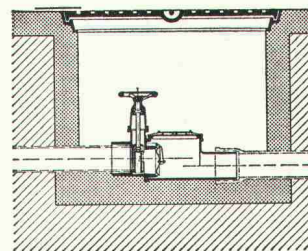
Rückstaudoppelschluss TRIPLEX für durch- gehende Leitungen
