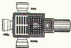
Kellerablauf «Junior» mit Rückstaudoppelschluss
