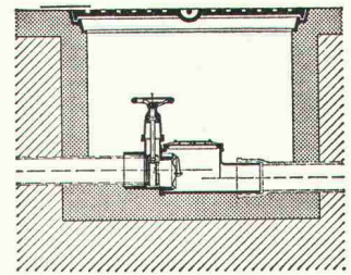
Rückstaudoppelschloss TRIPLEX für durch- gehende Leitungen
