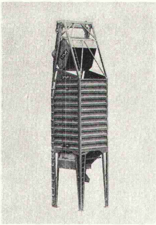
Betonieranlagen Kiessilos
