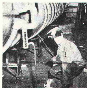
Klemmen (10 Tonnen)
