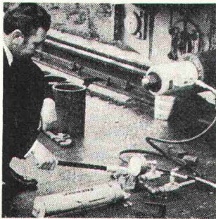
Vorspannen (60 Tonnen)
