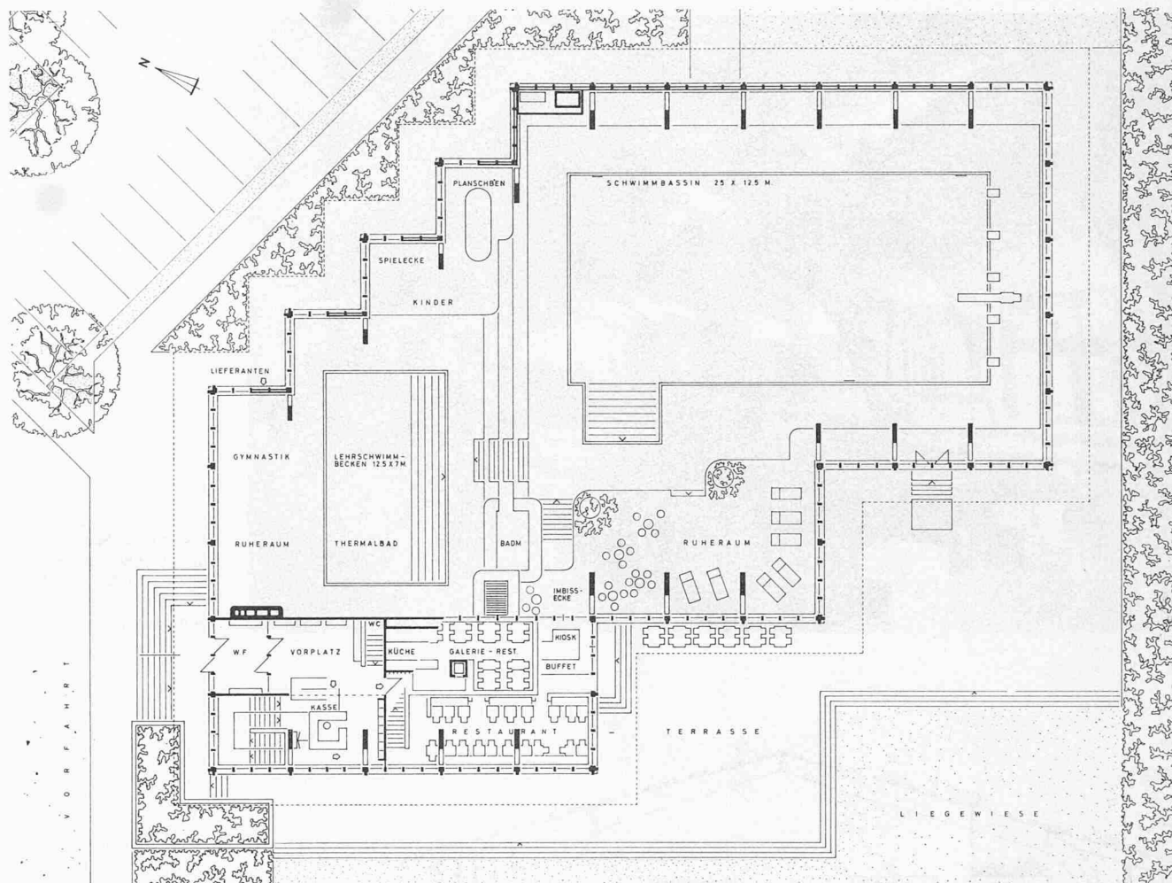
Hauptgeschoss 1:400
