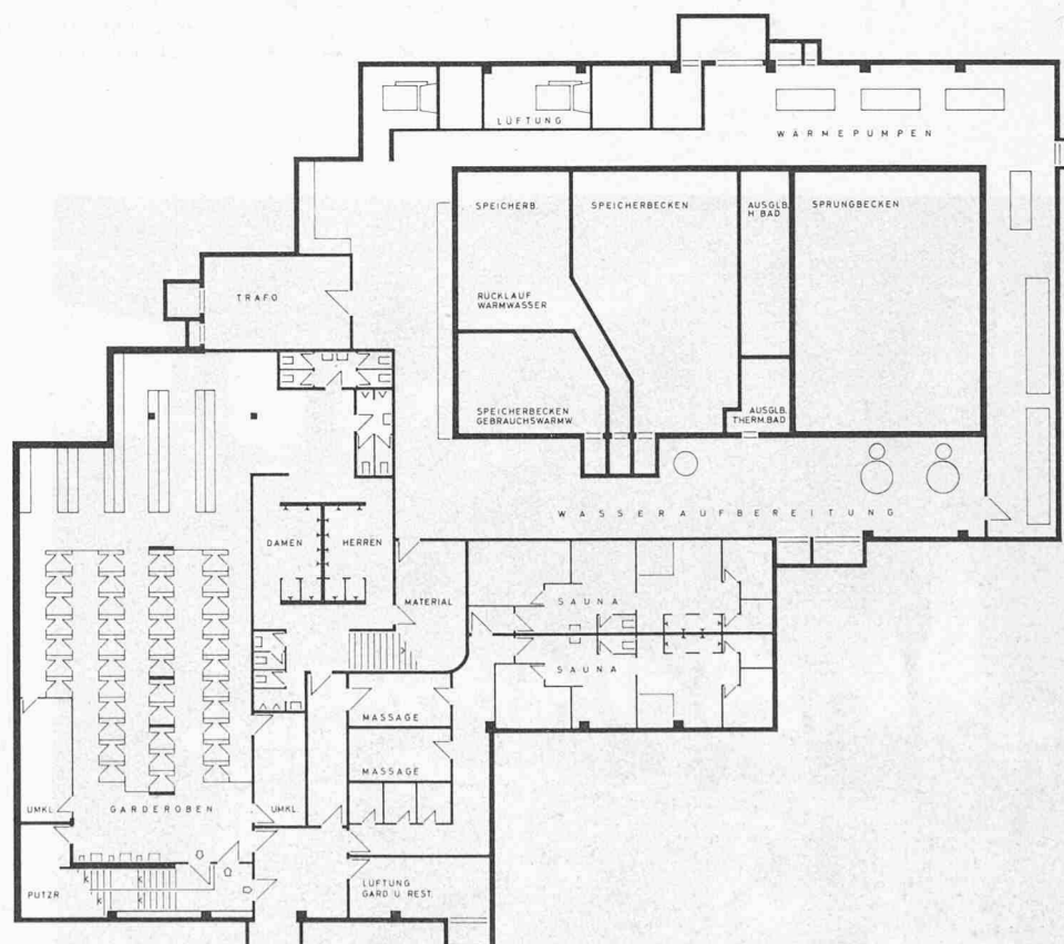
Untergeschoss 1:400
