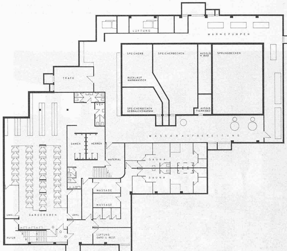
Untergeschoss 1:400
