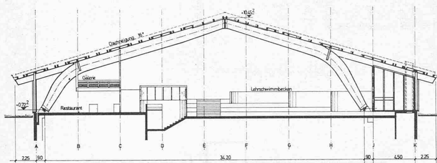
Querschnitt (Binderachse) durch Restaurant (Galerie) 1:400
