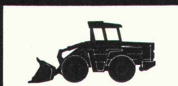
Radlader Europ L 2000 Motor: 185 SAE-PS Schaufeln: 1,6–3,6 m 3 Gewicht: 14.000 kg
