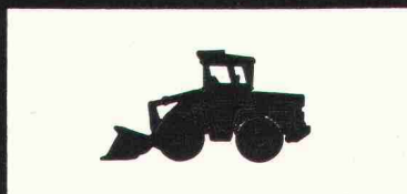
Radlader Europ L 800 Motor: 80 SAE-PS Schaufeln: 0,5–1,3 m 3 Gewicht: 6.000 kg
