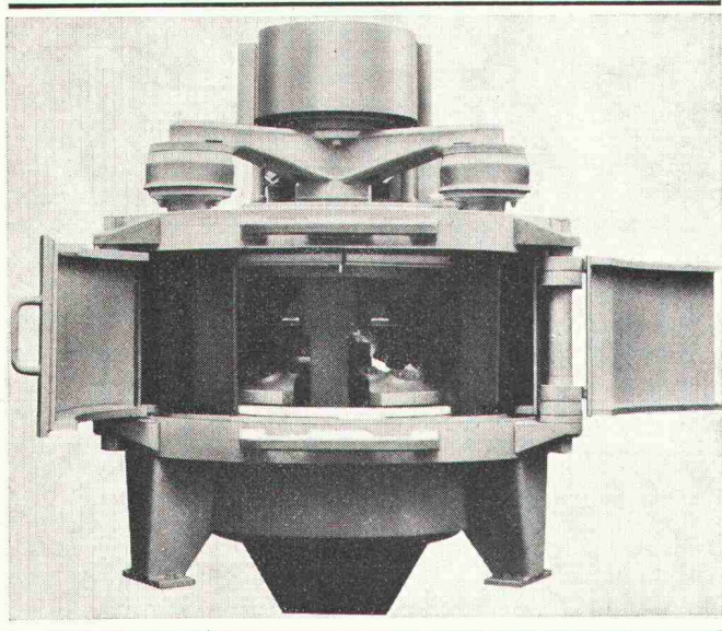
TURBO-Zentrifugal-Hammerbrecher Patent Pozzato
