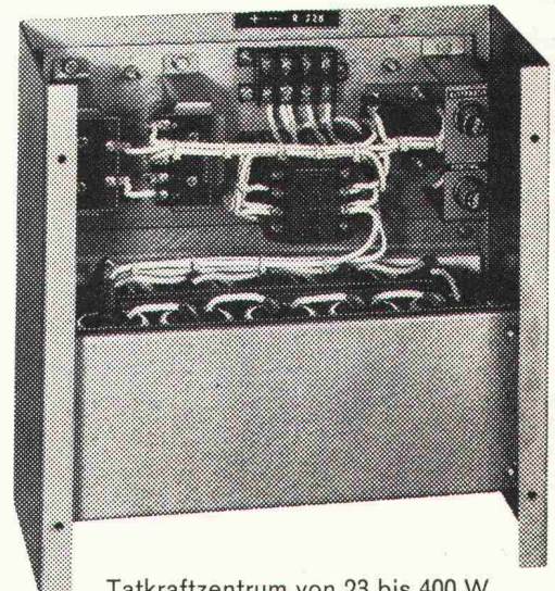
Tatkraftzentrum von 23 bis 400 W
