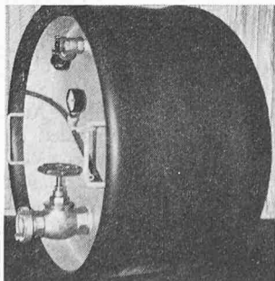
Eia-Abdrückelement im Ausgangszustand als Prüfgerät für die Dichtigkeit von Rohrleitungen und Kanälen
