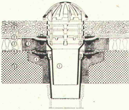
Kiesschüttdach, 2teilig
