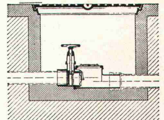
Rückstaudoppelschluss TRIPLEX für durch- gehende Leitungen
