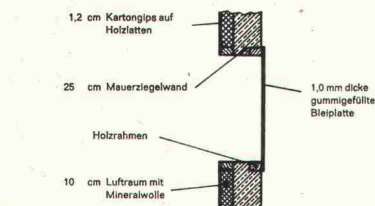
Aufbau des Prüfgegenstandes
