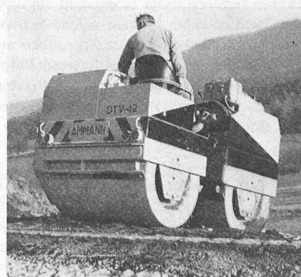
Bild 3. Doppel-Tandem Vibrationswalze DTV-42, Gewicht 4400 kg, Walzendurchmesser 920 mm, Walzenbreite 1230 mm, Mittelpunktklenkung-Doppelantrieb
