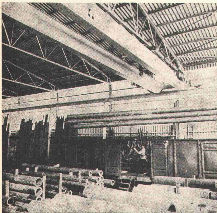
Bild 1. Moderner Zweiträger-Laufkran in Kastenbauweise
