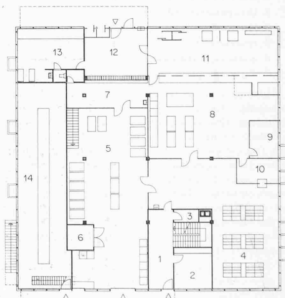
Erstes Obergeschoss 1:400. 1 Treppenhaus/Korridor, 2 Vorraum, 3 Betriebs-Montageraum, 4 Magazin, 5 Werkstatt, 6 Garderobe Damen, 7 Garderobe Herren, 8 Sanitär-Verteilung, 9 Zentrale, 10 Erweiterung (Zentrale)
