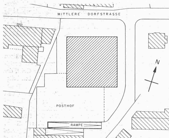
Oben: Lageplan 1:1000
