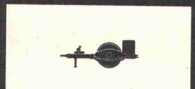
Vibrations-Anhängewalze VA 3 Statisches Gewicht: 3,3 t Arbeitsbreite: 2080 mm
