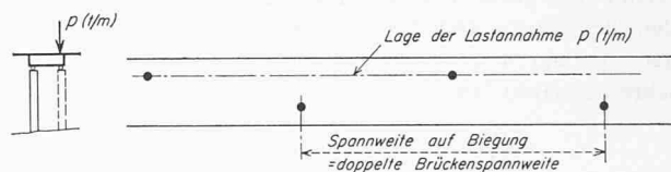
Bild 8. Anordnung der Stützen abwechselnd am äusseren Rand
