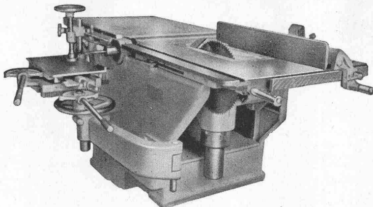
Universalmaschine HDU-50/60
