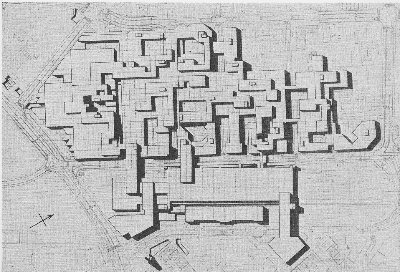
Lageplan 1:3500
