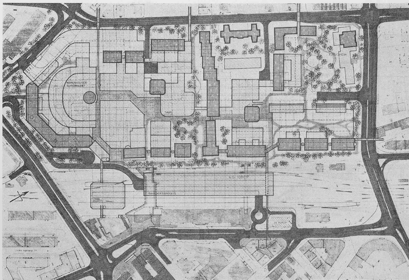
Lageplan 1:3500
