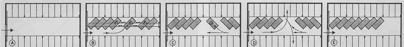
Bild 1. Parkieren in einer Garage mit zusätzlichen schräggestellten, längsverschiebbaren Drehplattformen. A Garage üblicher Bauart mit 24 ortsfesten Parkplätzen an beiden Längswänden. B in der gleichen Garage ist der Fahrstreifen durch sieben Rotex-Plattformen zusätzlich ausgenutzt. C soll ein Plattformparkplatz verlassen werden, so dreht sich die Plattform nach entsprechendem Drucktastenbefehl um 90°. D soll ein ortsfester Parkplatz an der Wand befahren werden, so verschieben sich die davor stehenden Plattformen und öffnen einen grossen Manövriertplatz. E Rotex-Anlage mit eng zusammengefahrenen Plattformen (Ausgangslage)
