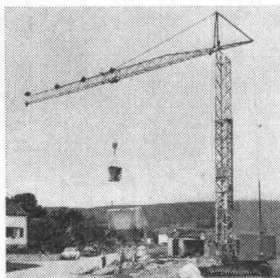
Laufkatzenkran Huggler H 20
