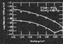
Fig. 14 Löslichkeitskurven und Antimonion in Schwefelsäure nach Ruetzsch und Angstadt (1)
